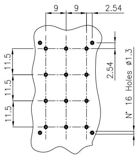
P.C.B. CUTOUT DIMENSIONS
